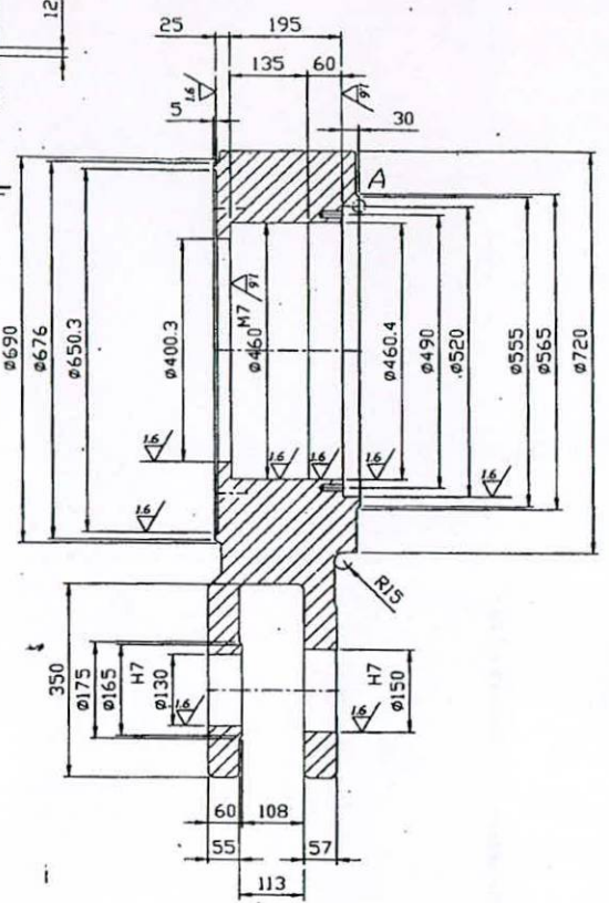
SEC A-A
